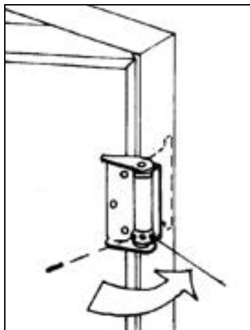
Portas com abertura para a ESQUERDA. O anel com furos esta para cima
